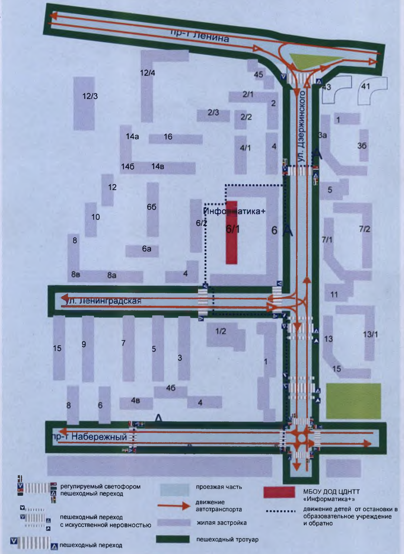
2. Схема организации дорожного движения в непосредственной близости от МБОУ ДОД ЦДНТТ «Информатика+» по адресу: ул. Дзержинского 6\1 с размещением соответствующих технических средств организации дорожного движения, маршрутов движения детей и расположения парковочных мест
