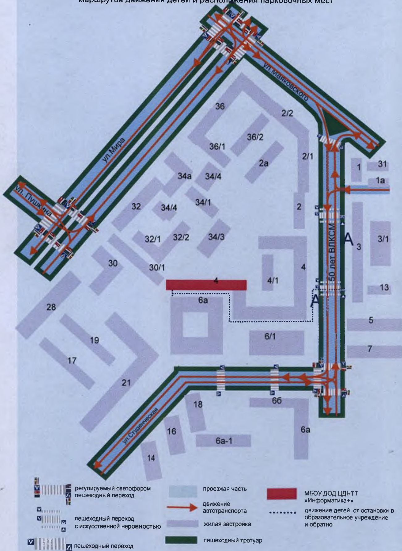
2. Схема организации дорожного движения в непосредственной близости от МБОУ ДОД УДНТТ «Информатика+» по адресу: ул. 50 лет ВЛКСМ 4 с размещением соответствующих технических средств организации дорожного движения, маршрутов движения детей и расположения парковочных мест
